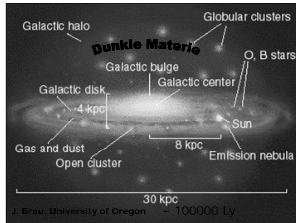
Schema der Struktur, Dimensionen und Komponenten der Milchstraße
