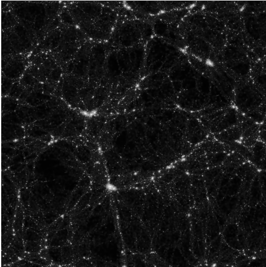
Computersimulation der Struktur des Universums Skala: 1 Milliarde Ly
